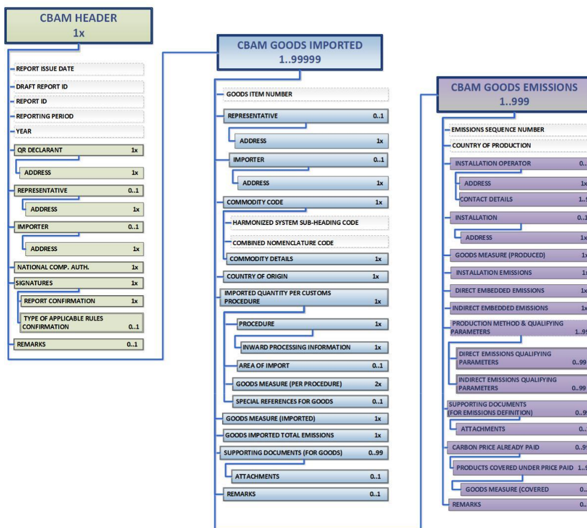
Slika 29: Podatkovni model CBAM izvješća
